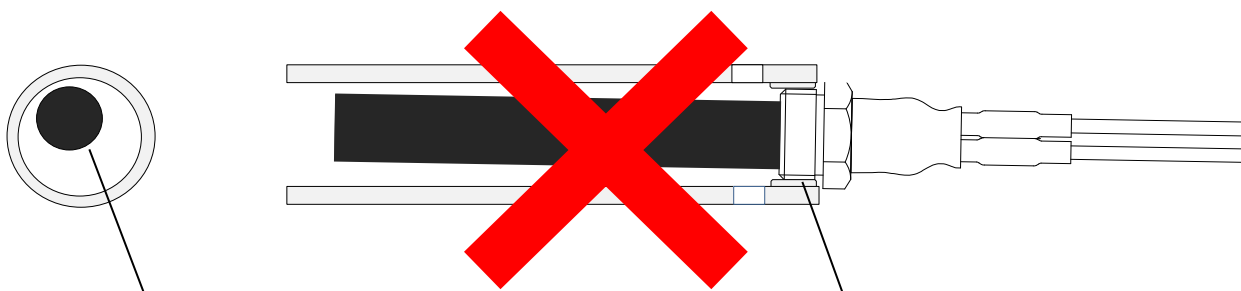
Elément chauffant incliné en raison d'un mauvais système de fixation ou mauvais filetage
