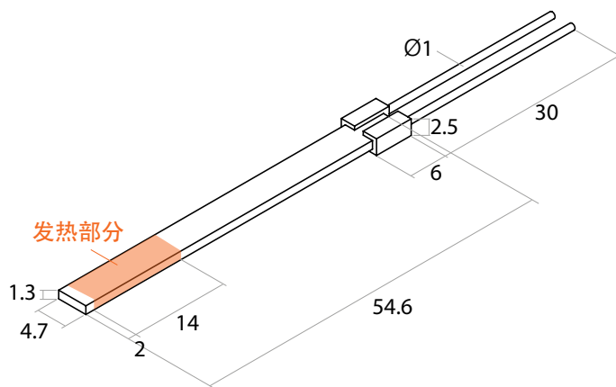
加热元件 54.6 mm
