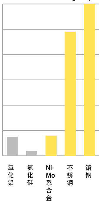
侵蚀减重 60% H 2 SO 4
