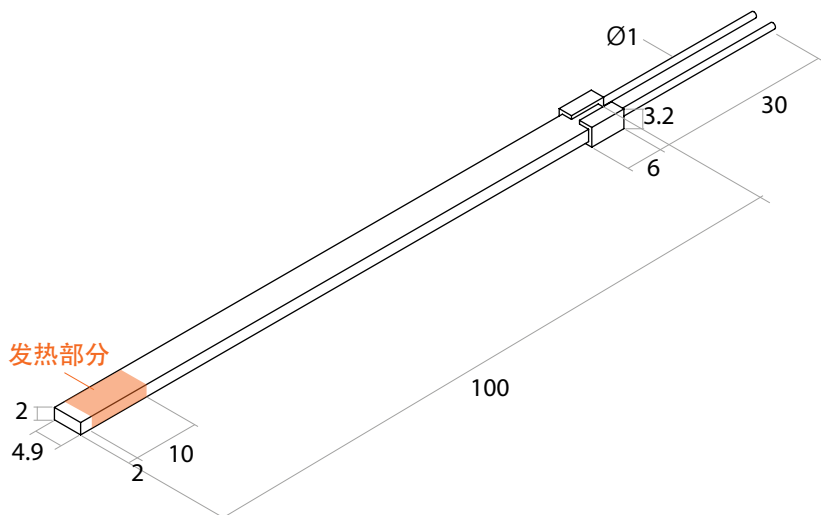
加热元件 100 mm
